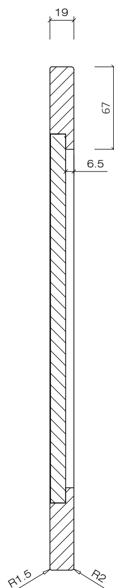
B-B
