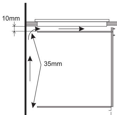
Aménagement dans le plateau d'un meuble porteur.
