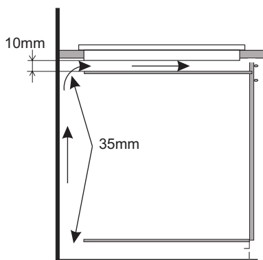
Einbau in der Arbeitsplatte des tragenden Schrankes.
