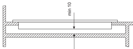
Einbau in der Arbeitsplatte des tragenden Schrankes.
