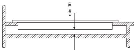
Aménagement dans le plateau d'un meuble porteur.
