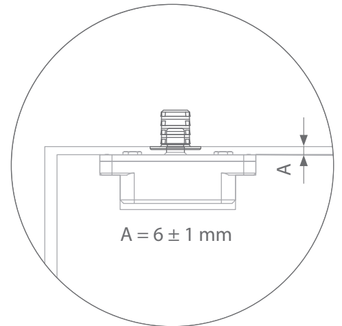
LINTEEL MONTAGE / MONTAGE SOUS LINTEAU / LINTEL MOUNT / MONTAGE IM STURZ / MONTAJE DINTEL
