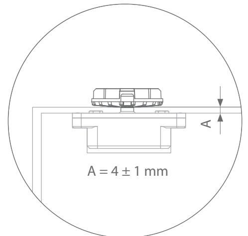
PLAFONDBEVESTIGING / MONTAGE AU PLAFOND / CEILING MOUNT / DECKENMONTAGE / FIJACIÓN EN TECHO
