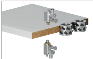
1 Formatierungszone
