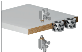
1 Voorfreesunit
