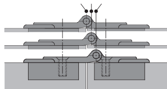
Draaipuntverschuiving 0 3 6 mm
