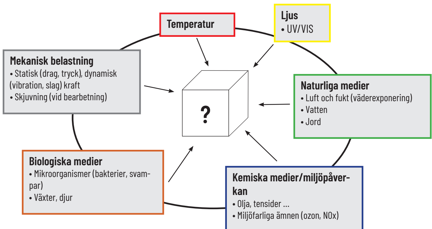
Figur: Belastningar på polymaterial, källa: prof. dr Samuel Affolter, Langzeitverhalten von Thermoplasten, Interstaatliche Hochschule für Technik, Buchs, Schweiz, figur 1, sida 3
